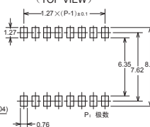
印刷基板加工尺寸 (TOP VIEW)
